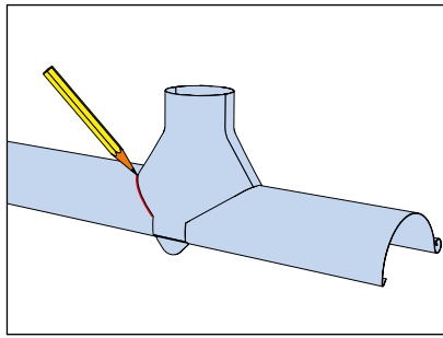
2. Den Rinnenablauf als Schablone benutzen.
