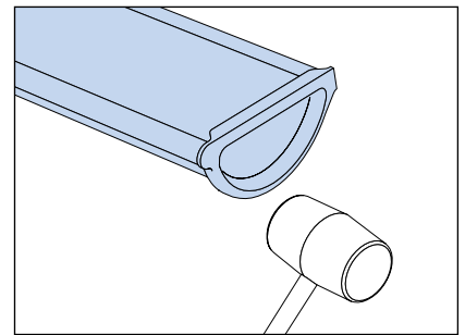
8. Das Endstück RG ist selbstdichtend. Es ist am Ende der Rinne zu befestigen und leicht mit einem Gummihammer zu befestigen. Achtung! Bei der Verwendung von Rinneneisen, wo die Rinne an ihrem Platz festgeklemmt wird, sollte das Endstück erst befestigt werden, wenn die Rinne in den Rinnenhaltern befestigt worden ist.
