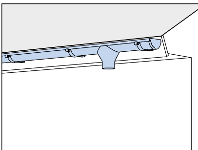
9. Die Rinne ist in den Rinnenhaltern zu befestigen und die Rinne ist beim Loch für den Rinnenablauf zu biegen, so dass auf beiden Seiten in Richtung zum Rinnenablauf Gefälle ist.
